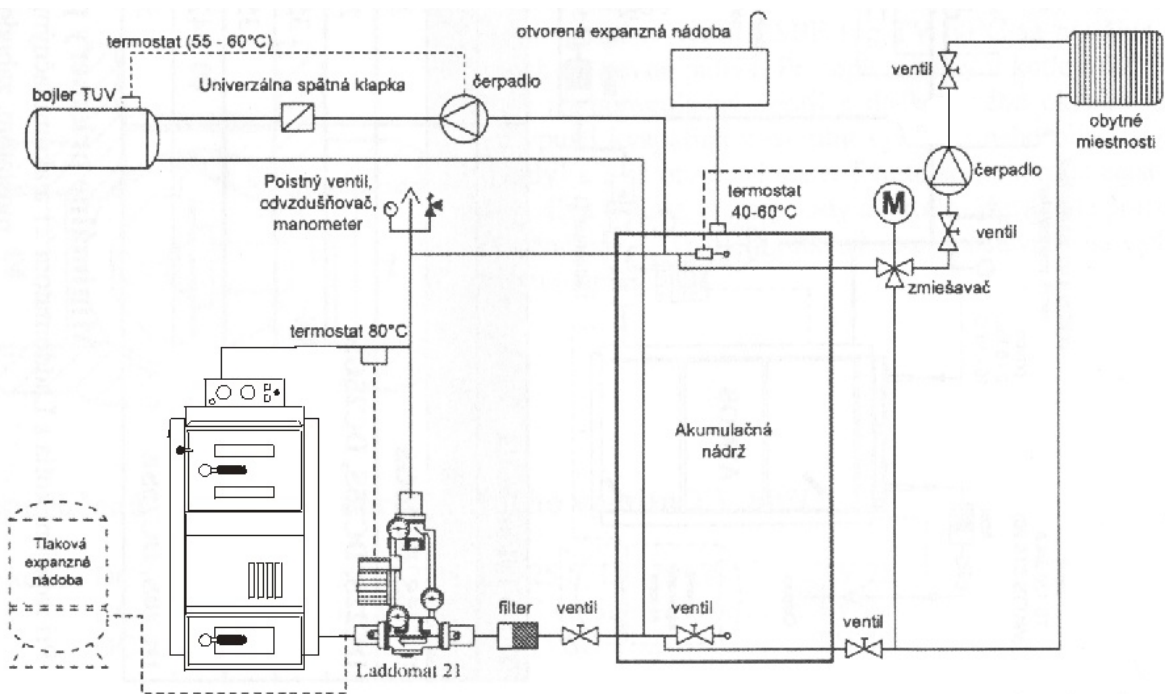
Zapojenie kotla s akumuláčnou nádržou
