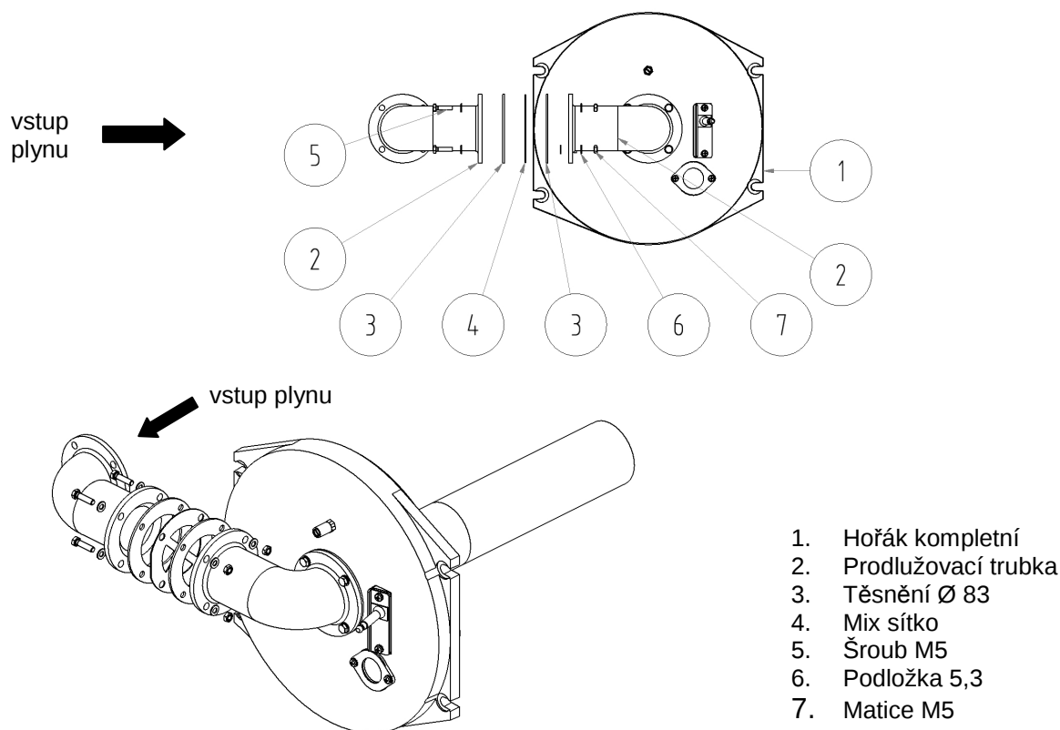
Obr. č. 3 Umístění mix sítka v plynové větvi hořáku K 2 L5X
