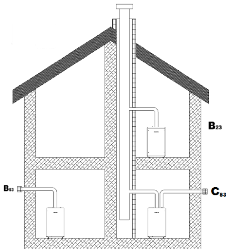
Obr. č. 11 Možnosti připojení odtahu spalin a přívodu vzduchu
