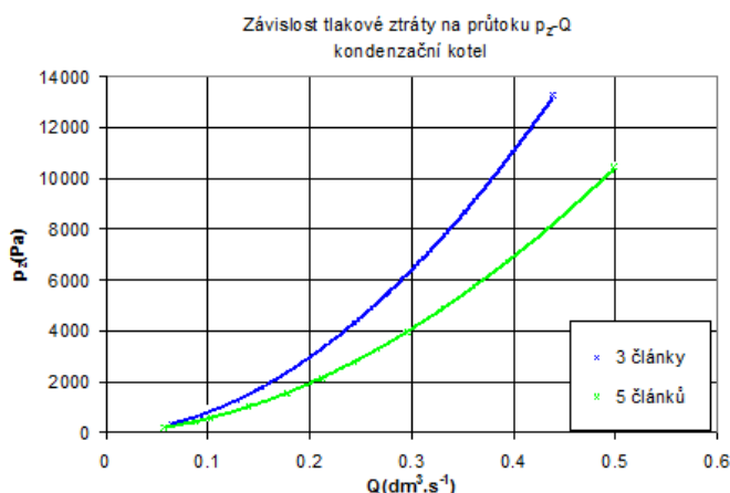
Obr. č. 1 Závislost tlakové ztráty na průtoku
